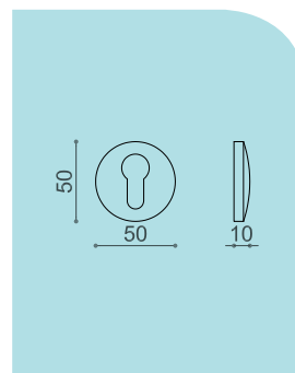
BOCCHETTA_ESCUTCHEON
