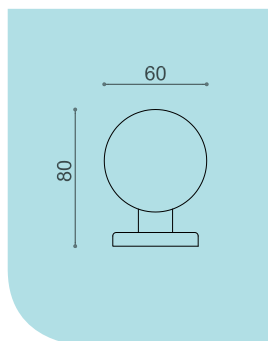
POMOLO_KNOB
