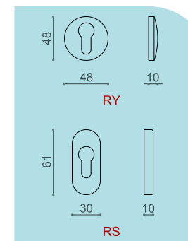
BOCCHETTA_ESCUTCHEON
